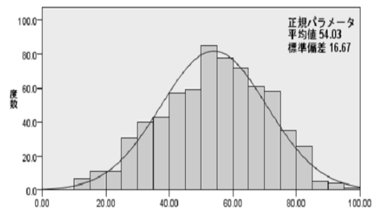
(5-16図) 百分換算点の KS 正規分布検定
