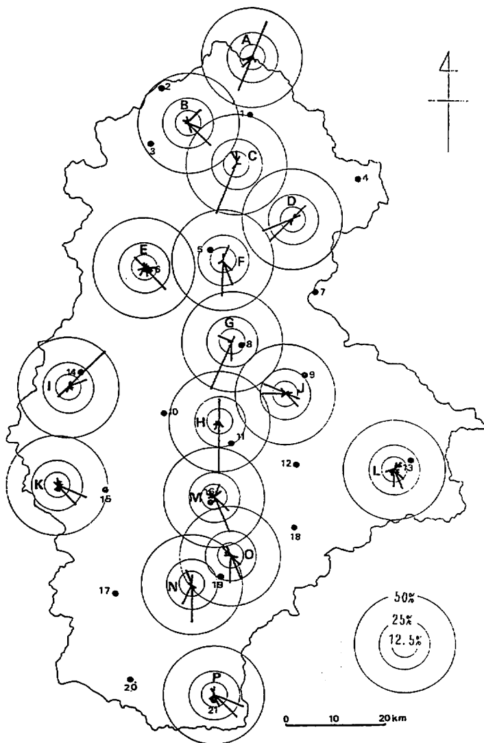
図3 各地点における日最多風向頻度図 (%) (1988.8.9~9.8)
