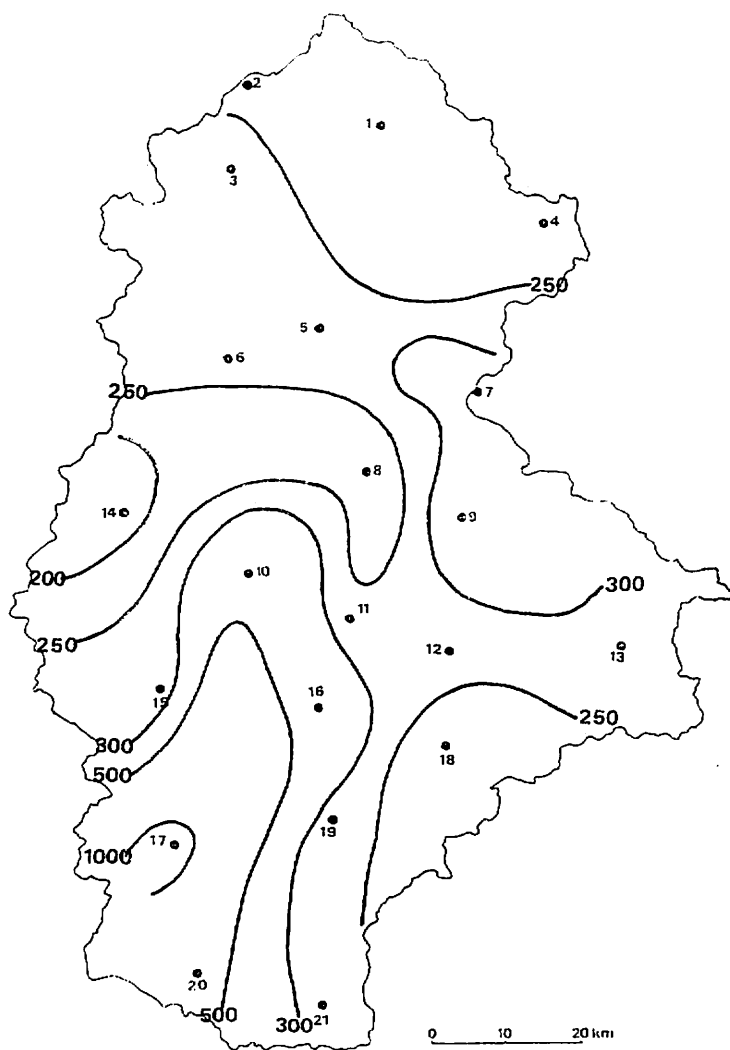
図2 調査期間中における降水量分布図 (mm) (1988.8.9~9.8)
