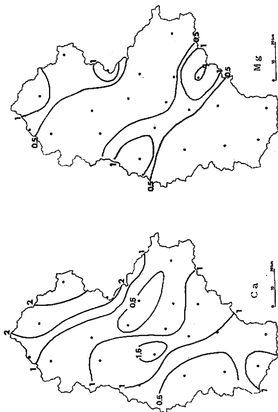
図4-3 各成分ごとの等降下量線図 ( \mu\text{g}/\text{km}^2/\text{day} )
